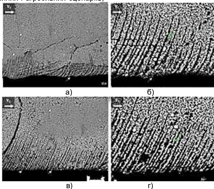
Рис. 7. Мікроструктурна цілісність поверхні в результаті звичайних умов різання; а – опір матеріалу, спричинений проміжними тепловими ефектами та механічними впливами низької інтенсивності; б – деталі слідів деформації, спричинених термічними ефектами низької інтенсивності та проміжними механічними впливами на поверхні заготовки; в – опір матеріалу, викликаний помірними тепловими ефектами та проміжними механічними впливами; г – деталі слідів деформації, спричинених помірними термічними та проміжними механічними впливами.
