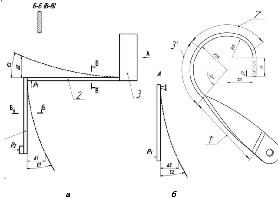
Рисунок 3 - Розрахункова схема до обґрунтування конструкції стояка
