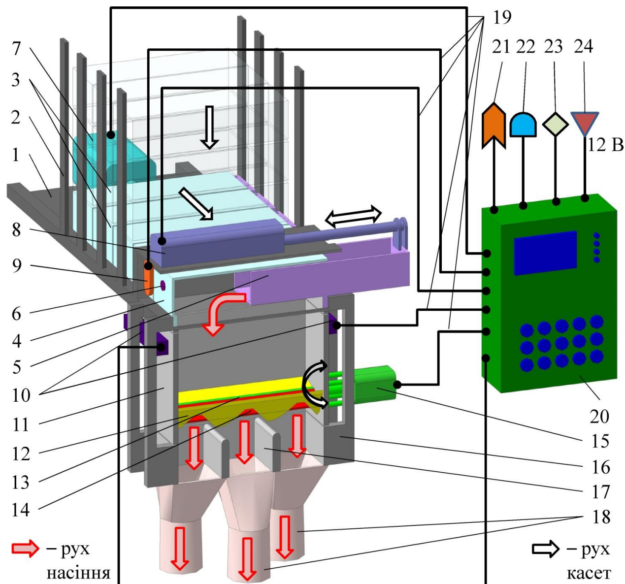
Рис. 4. Конструктивно-технологічна схема висівного апарата селекційної сівалки дрібнонасінневих культур
