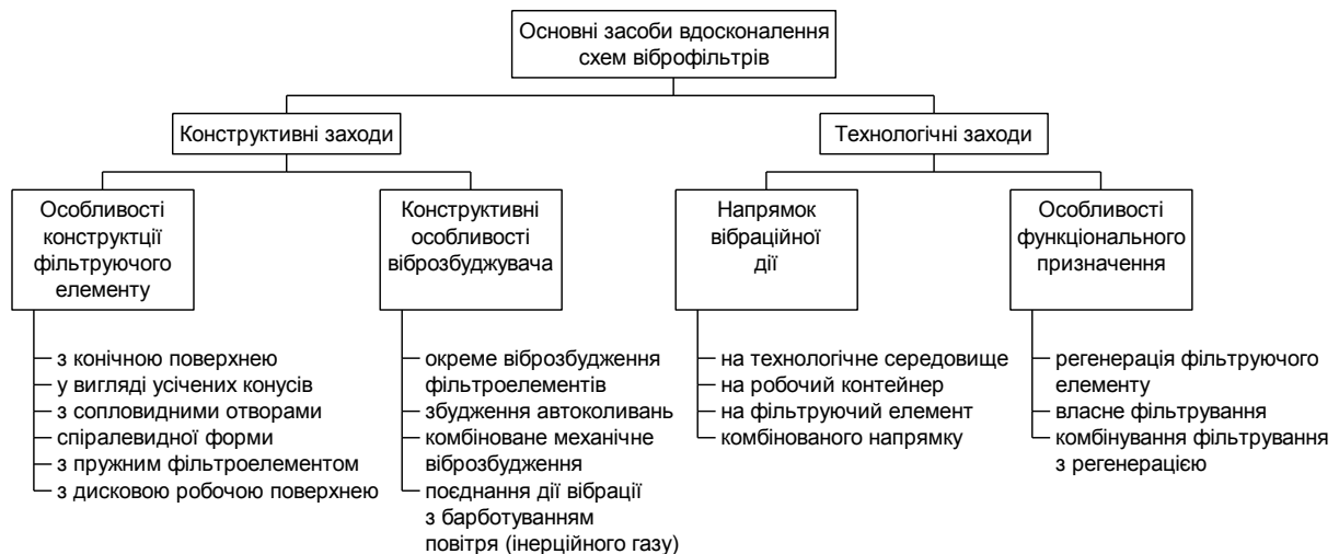
Рис. 8. Основні засоби вдосконалення конструктивних та технологічних схем вібраційних фільтрів
